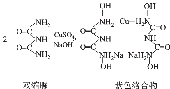
图 2-3 双缩脲反应图示
