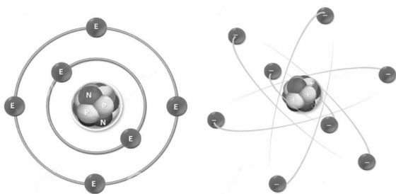
图 2-2 碳原子的电子结构示意图
